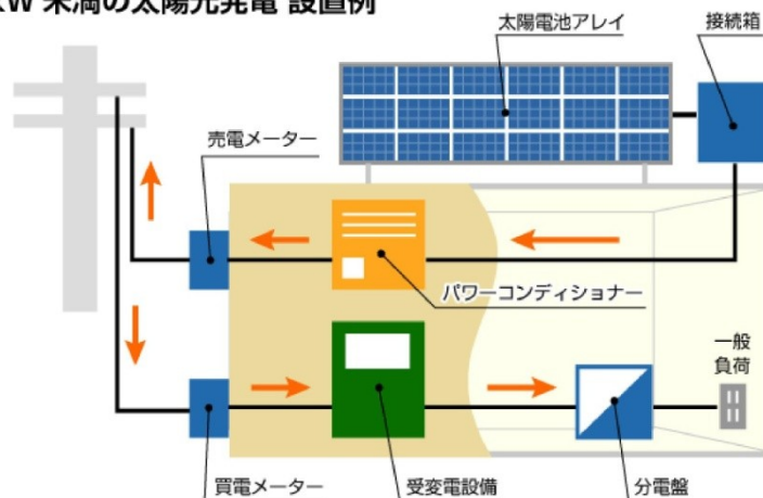
50kW未満の太陽光発電 設置例
